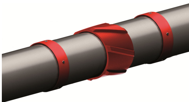
Рис. Центратор стальной жесткий спиральнолопастной тип 513
