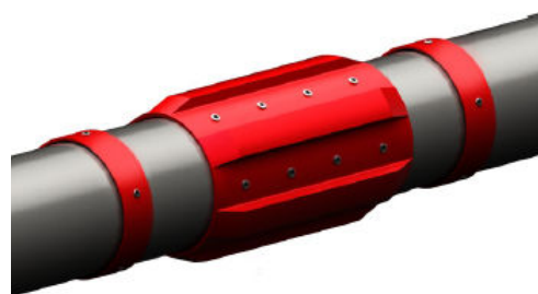
Рис Центратор алюминиевый жесткий прямолопастной тип 531
